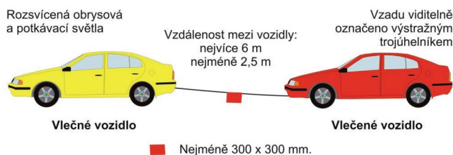
Ilustrační obrázek – vlečení vozidel na laně:
